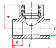
Тройник комбинированный ВР
