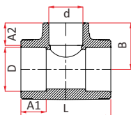
Тройник переходной
