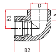
Угол 90° комбинированный ВР
