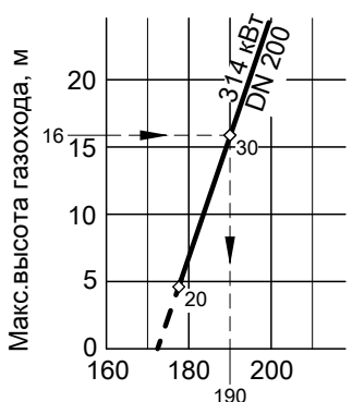
Необходимый общий напор горелки, Па
