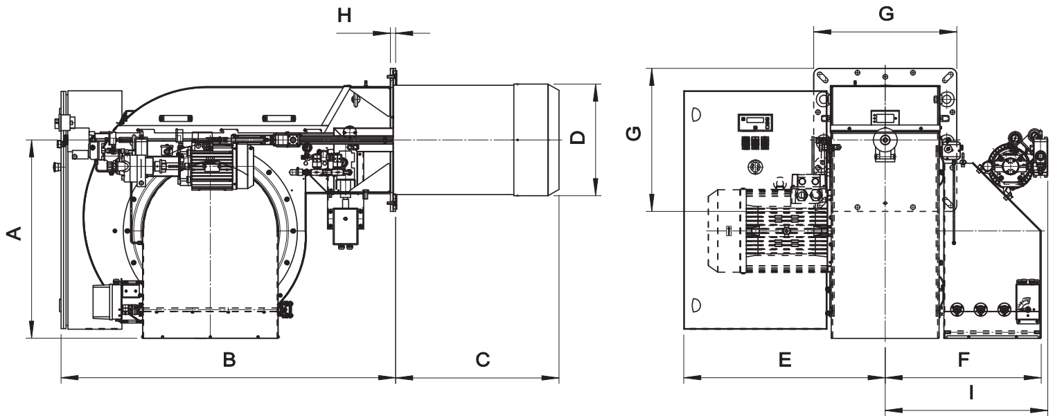
Fig. 2 Burner dimensions
