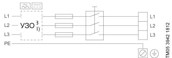
Рис. 74. Пример электродвигателя, подключенного к сети, с сетевым выключателем, плавким предохранителем, допускающим отстройку от пускового тока, и дополнительной защитой
