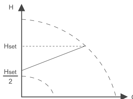
Рис. 37. Пропорциональное давление
