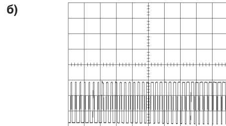
Рис. 81 а) ток электродвигателя и напряжение б) участок напряжения электродвигателя
