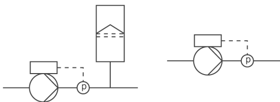
Рис. 40. Постоянное давление
