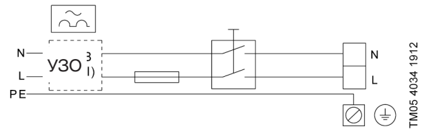
Рис. 73. Пример электродвигателя, подключенного к сети, с сетевым выключателем, плавким предохранителем, допускающим отстройку от пускового тока, и дополнительной защитой
