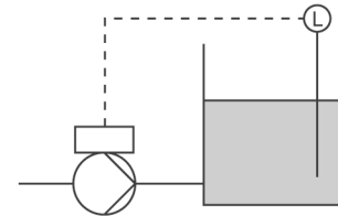
Рис. 50. Постоянный уровень
