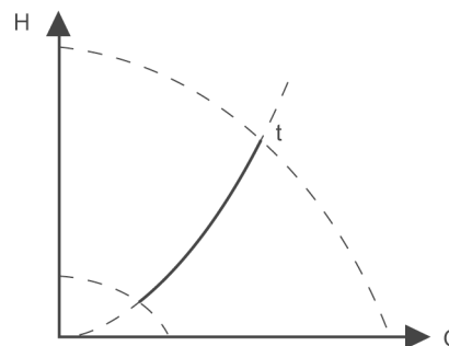
Рис. 41. Постоянная температура
