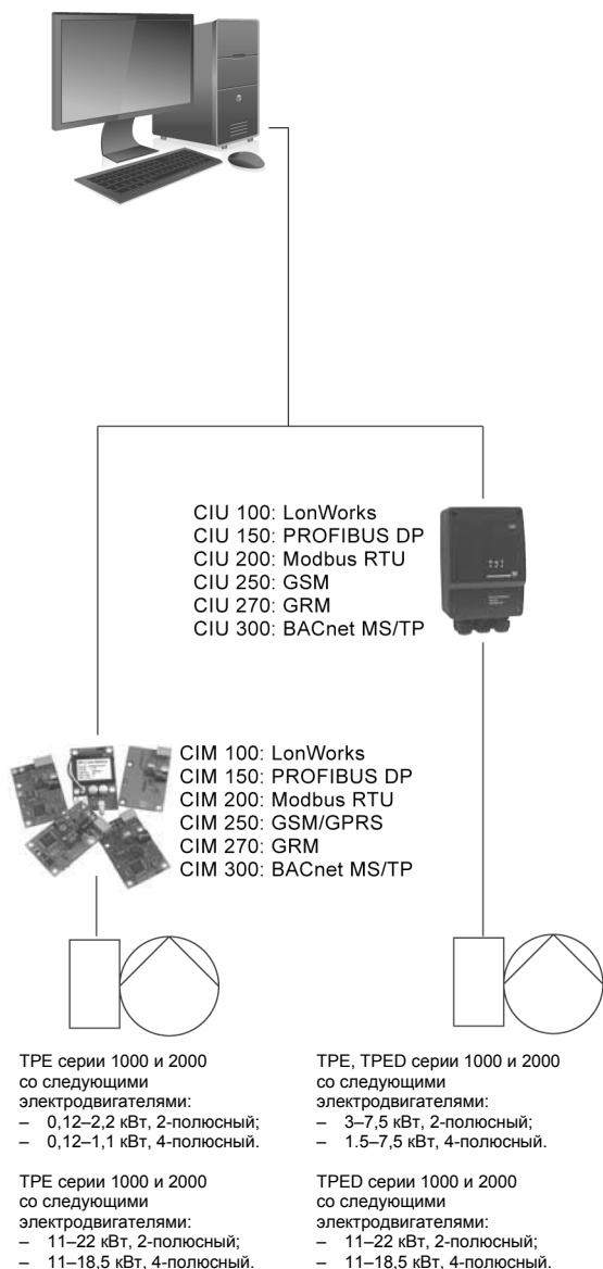
Рис. 65. Структура центральной системы управления зданием
