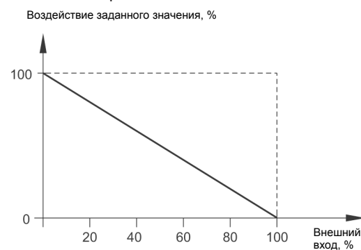
Рис. 57. Обратная функция
