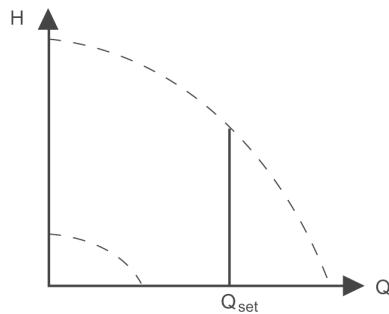
Рис. 47. Постоянная подача
