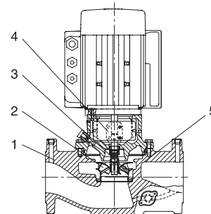
Рис. 68. Разрез однофазного насоса TP серии 200 (с фланцевым присоединением)
