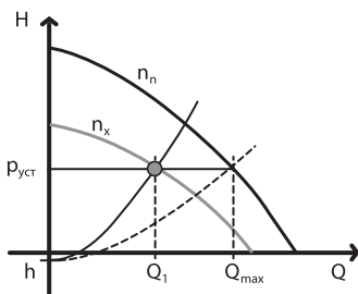
Рис. 7 Регулирование по постоянному давлению
