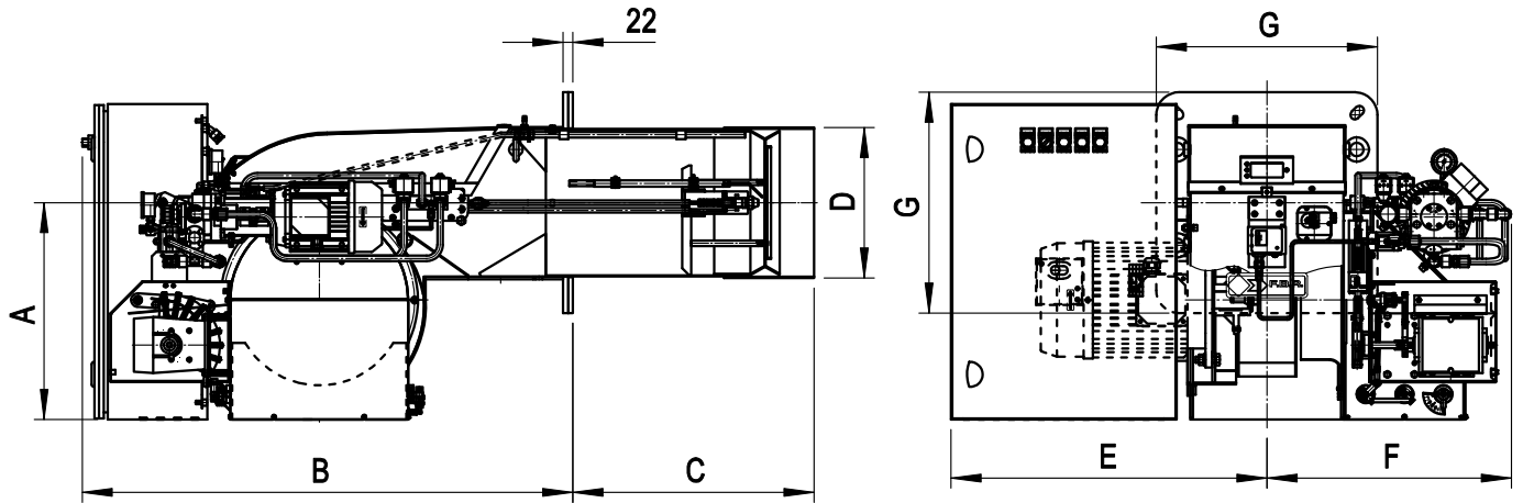
Fig. 3 Dimensions FGP 350/M - FGP 450/M - FGP 550/M
