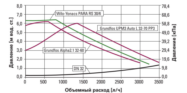
Насосная группа со смесителем K32 DN32
