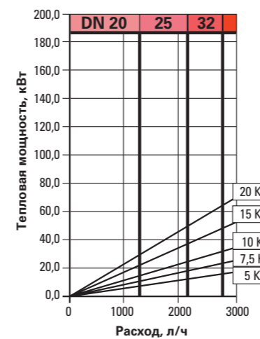
Насосная группа прямого контура K31
