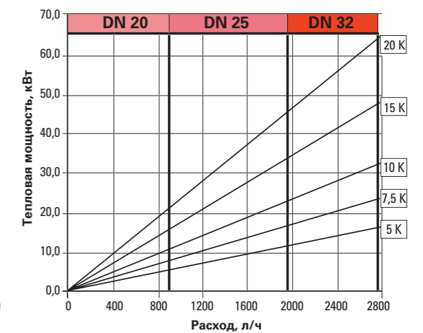
Насосная группа со смесителем и байпасом K34
