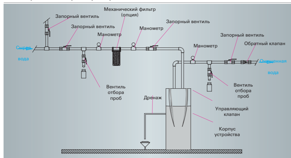
Схема установки фильтра Aquacarbon
