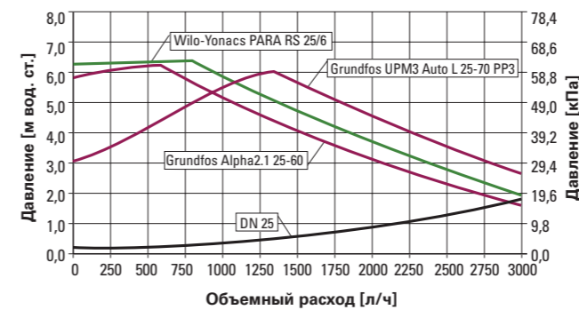
Насосная группа без смешения K31 DN25
