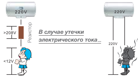
Водонагреватель с функцией Shock Proof
